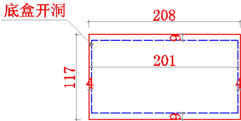
四联面板
