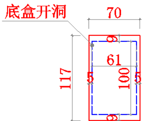
单联面板
