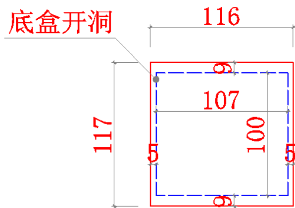
双联面板
